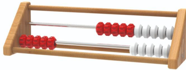
Rekenrek
